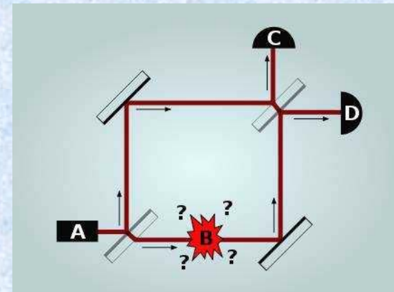
Elitzur-Vaidman bomb tester
